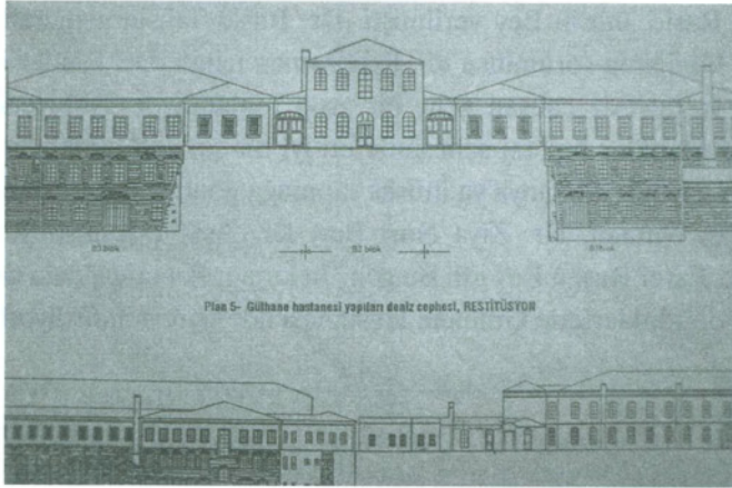
Gülhane Askeri Tatbikat Mektebinin Dulhane bölümünün planları
