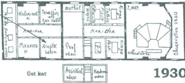
(ŞEKİL 12) Yeni projemizde teminini teklif ettiğimiz tesisat planı
